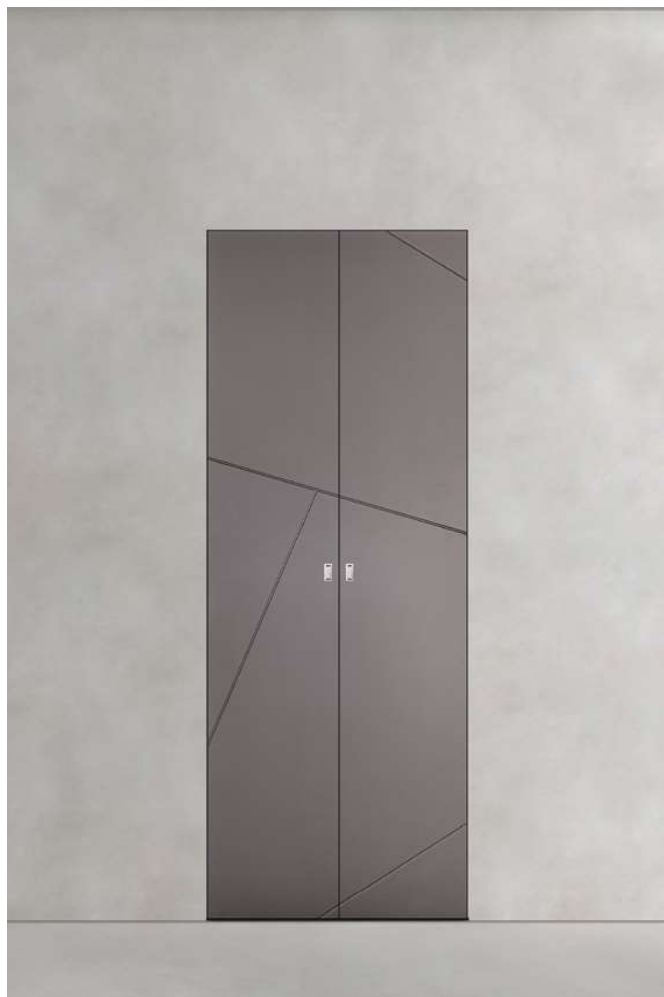
Armadio Modello: 603 due ante wall Finitura: Pirite Essenza: HDF (20 mm) Telaio: Legno + Alluminio Dimensioni: L 35cm + 35 cm x H 210 cm
