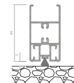
Libero sotto da 60 mm con spazzolino (a richiesta)
