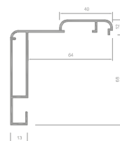
Telaio Z64 New
