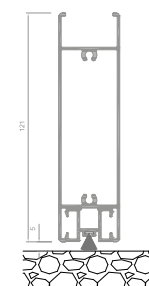
Libero sotto con spazzolino (a richiesta)
