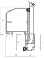
Anta battuta 17.5 (guarnizione laterale compatibile con i sistemi senza telaio, e per altri specifici telai tra cui telaio Trentino, Ghost e 264 New).
