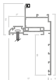
Telaio Z75 con distanziatore
