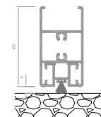
Libero sotto da 60 mm con spazzolino (a richiesta)
