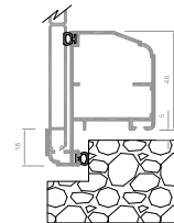
Anta battuta marmo (a richiesta)
