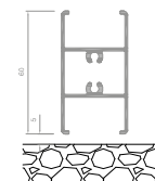
Libero sotto da 60 mm (a richiesta)
