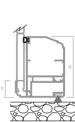
Anta a L (standarda)
