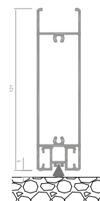
Libero sotto con spazzolino (a richiesta)
