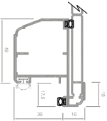
Anta battuta 17.5 (guarnizione laterale compatibile con i sistemi senza telaio, e per altri specifici telai tra cui telaio Trentino, Ghost e 264 New).
