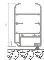
Anta a L (a richiesta)
