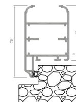
Anta battuta marmo (a richiesta)
