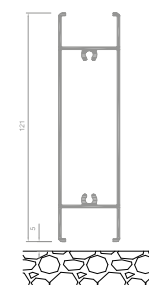
Libero sotto (standard)
