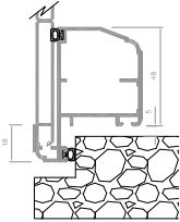
Anta battuta marmo (a richiesta)
