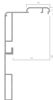
Telaio Z64 New con imbottito
