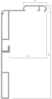
Telaio 264 New con imbottito
