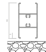
Libero sotto da 60 mm (a richiesta)
