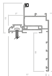
Telaio Z75 con distanziatore
